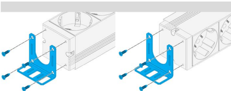
Haltewinkel montieren (4 Schrauben)
