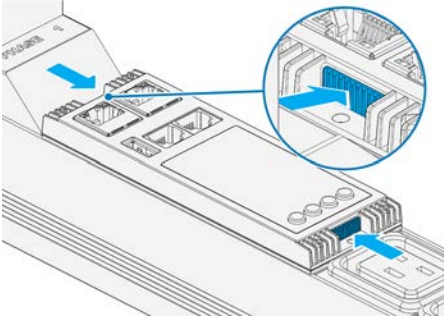
Rastrnasen eindrücken
