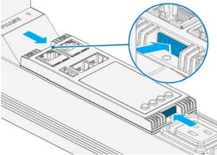
Rastrnasen eindrücken
